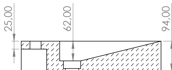
PRZĘKRÓJ G-G SKALA 1 : 7
